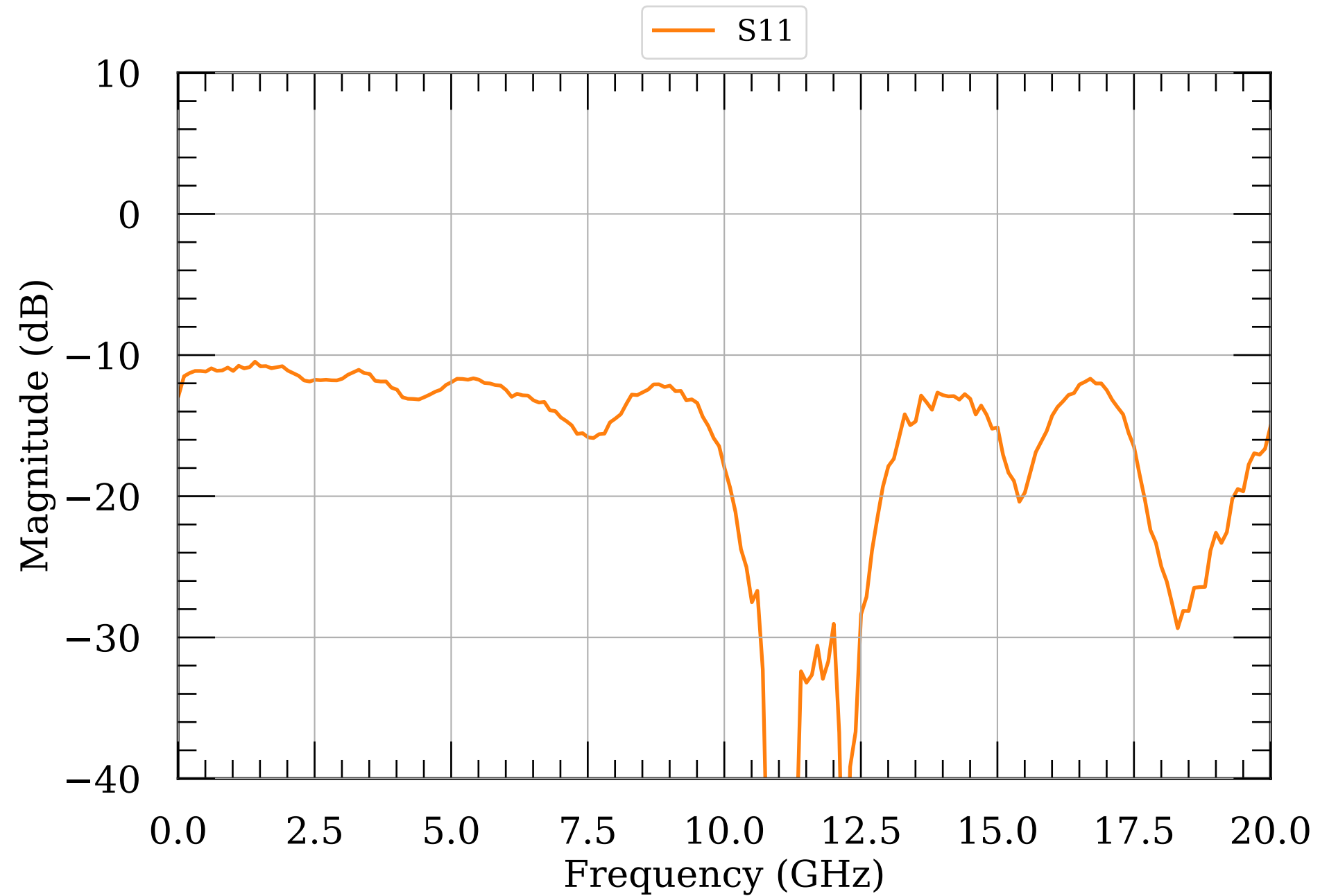
LNA S-params module087v2
